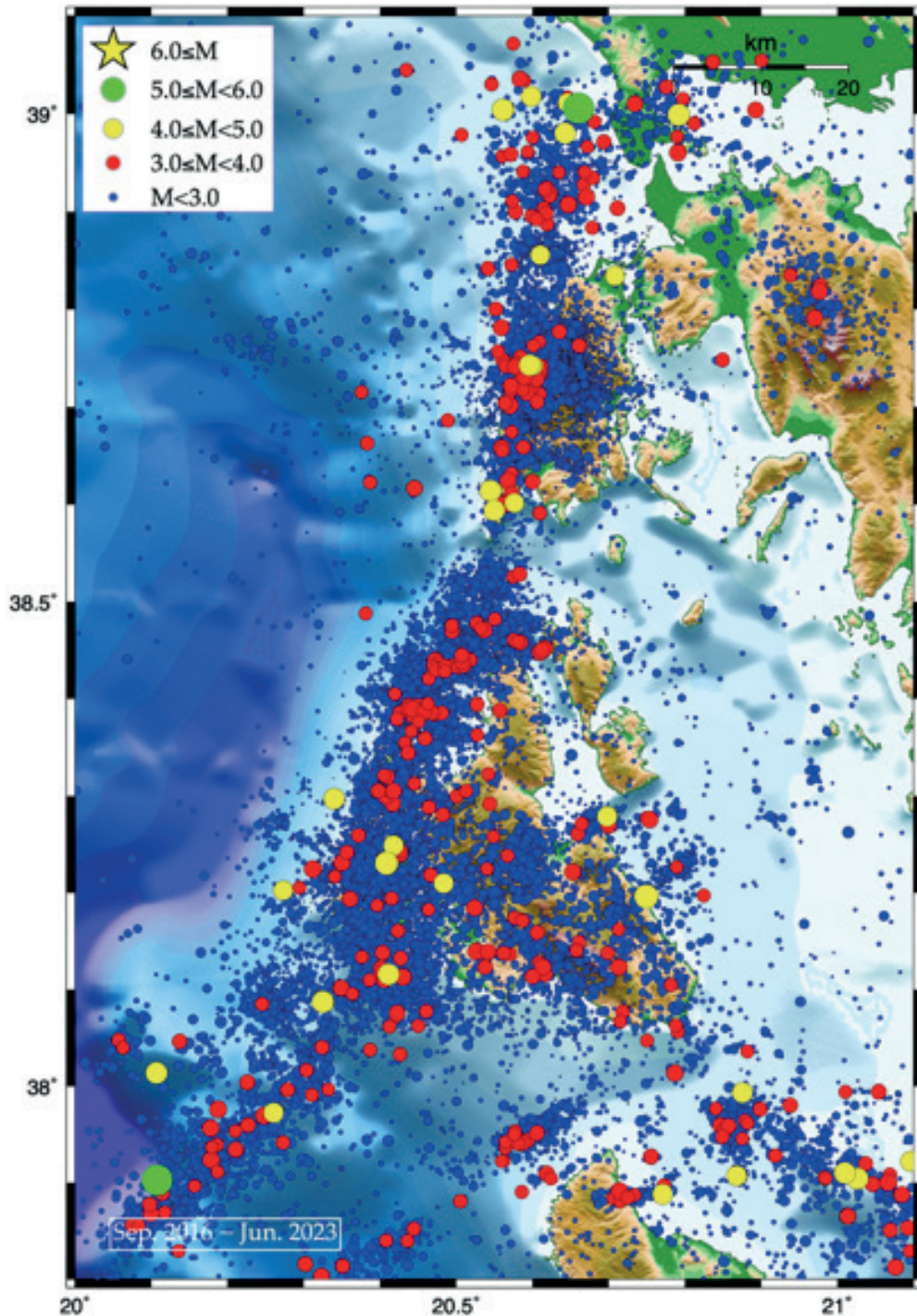
Σχ. 1. Κατανομή των επικέντρων των σεισμών που έγιναν στο χρονικό διάστημα Σεπτέμβριος 2016 - Ιούνιος 2023 στην περιοχή των κεντρικών Ιονίων Νήσων όπου για τον υπολογισμό των εστιακών τους παραμέτρων χρησιμοποιήθηκαν οι καταγραφές στο σεισμολογικό δίκτυο της ΠΕΔ-ΙΝ.
